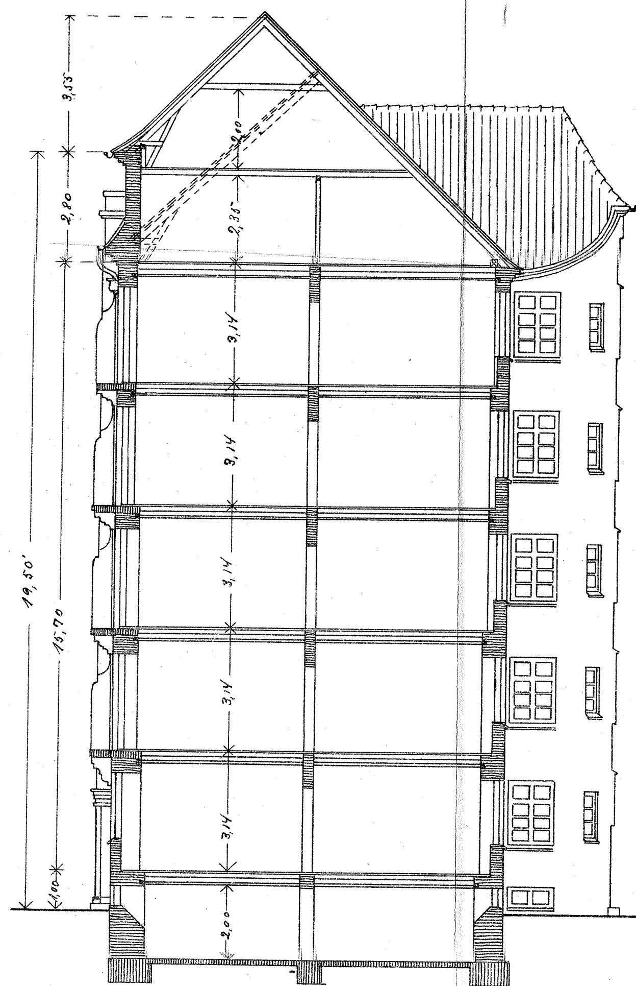
SNIT Gennem MIDPARTI MOD EJDERSTEDG.
